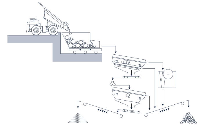
Master: Bei mäßigem Vorkommen kann Steinerde gezielt auf einer zweiten Siebmaschine abgeseibt werden. Die wertvollen Gesteinskörnungen werden der Produktion zugeführt und nur das ungeeignete erdige Material auf Halde abgeschieden.
